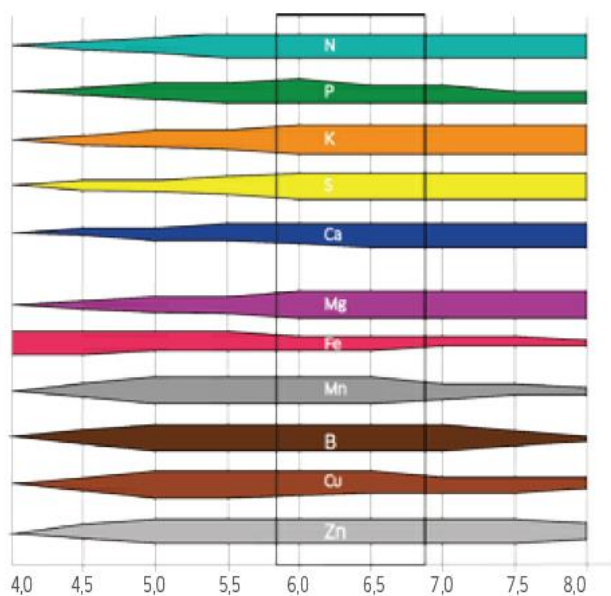
Jordens pH-værdi
